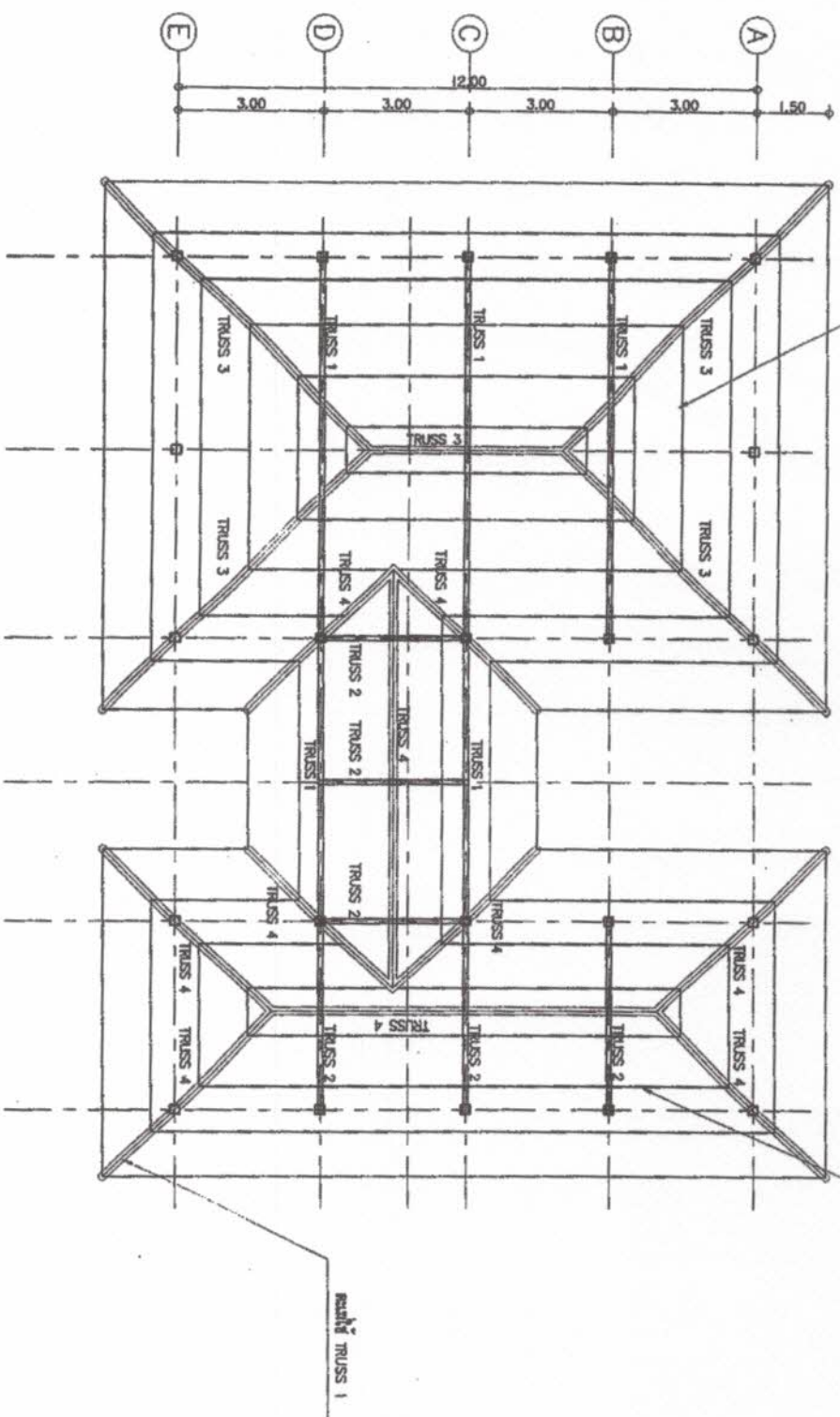
แบบโครงสร้างหลังคา (TRUSS) ขนาด 1 : 100
